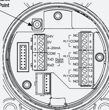
Terminal Module
